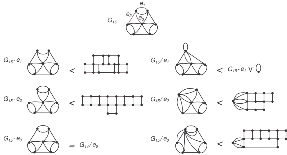
Fig. 16. G_{15} - e_i, G_{15}/e_i .
