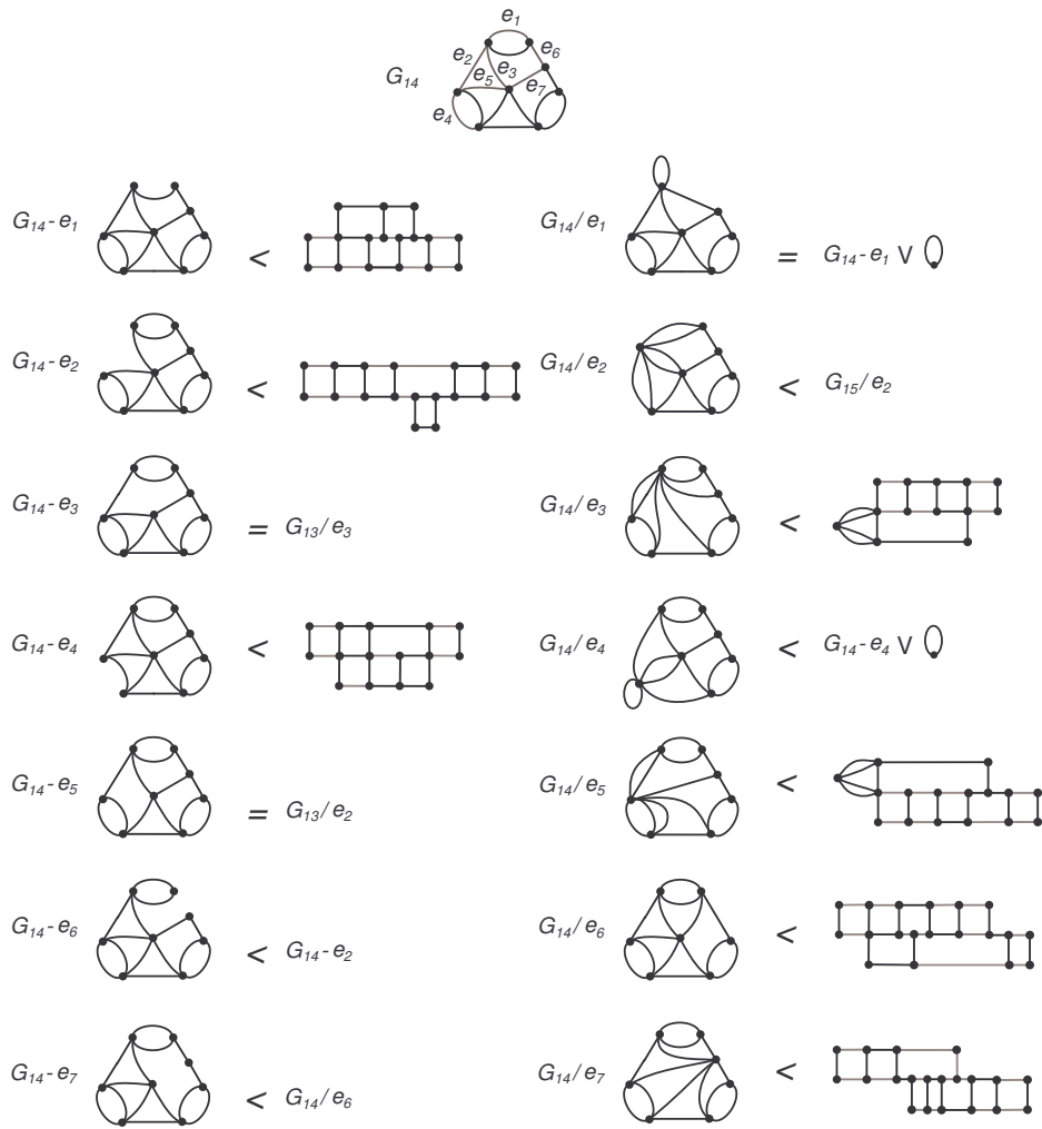
Fig. 15. G_{14} - e_i, G_{14}/e_i .
