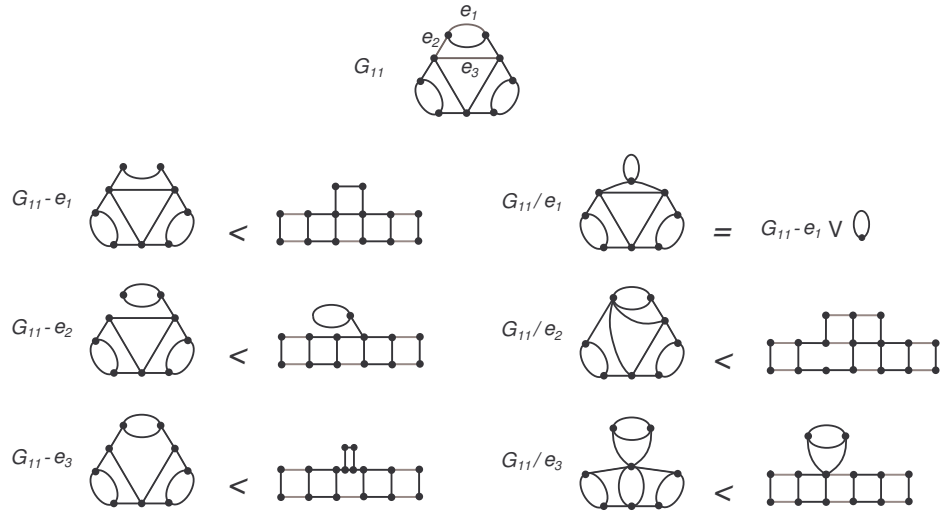
Fig. 12. G_{11} - e_i, G_{11}/e_i .
