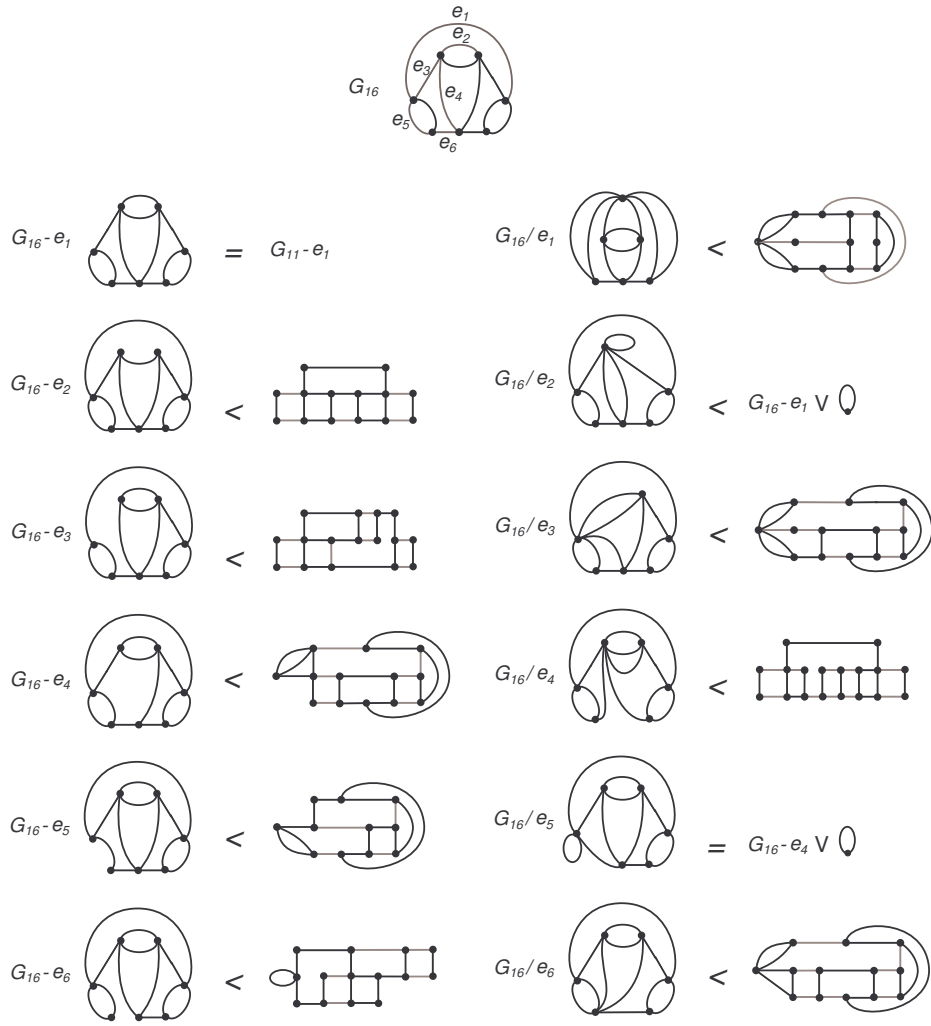
Fig. 17. G_{16} - e_i, G_{16}/e_i .
