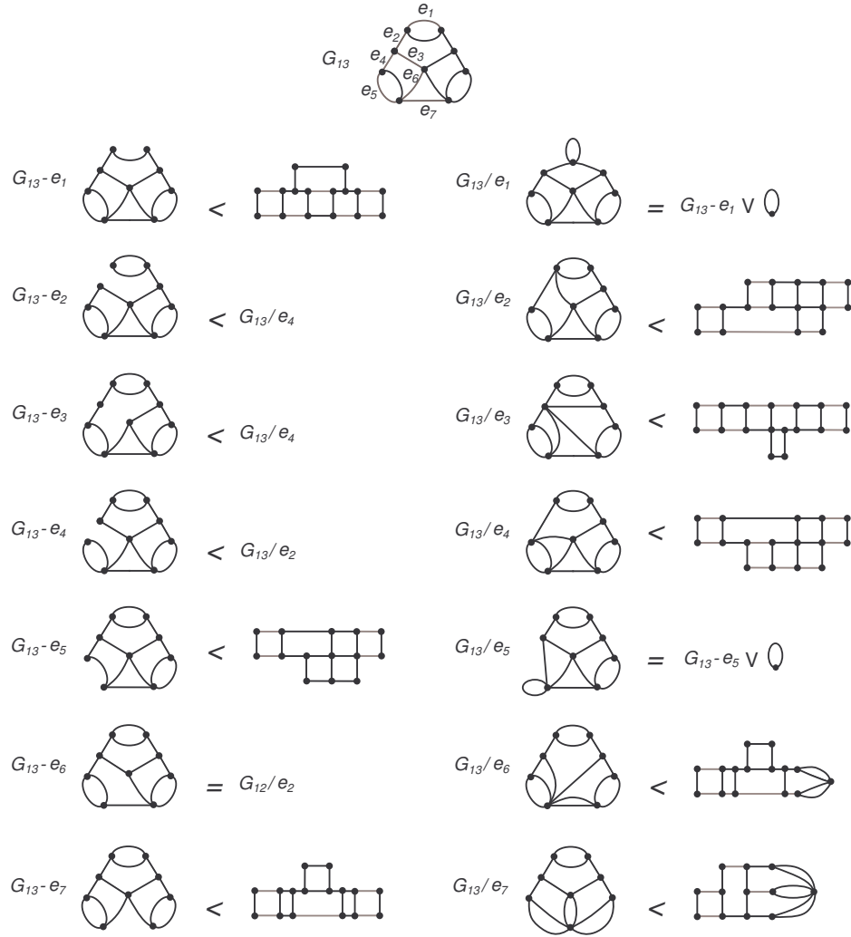
Fig. 14. G_{13} - e_i, G_{13}/e_i .
