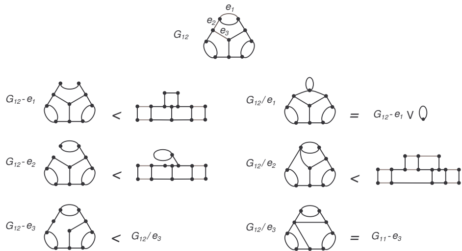
Fig. 13. G_{12} - e_i, G_{12}/e_i .
