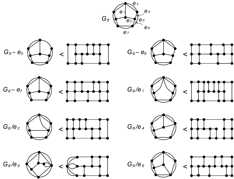
Fig. 9. G_8 - e_i, G_8/e_i .
