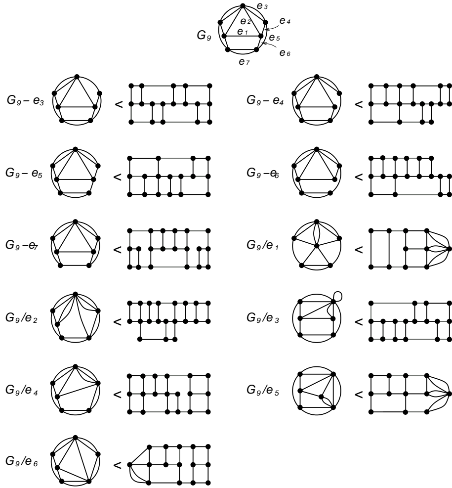
Fig. 10. G_9 - e_i, G_9/e_i .
